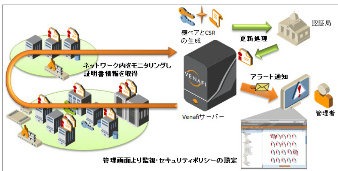
図) Venafi Encryption Director の各種機能
